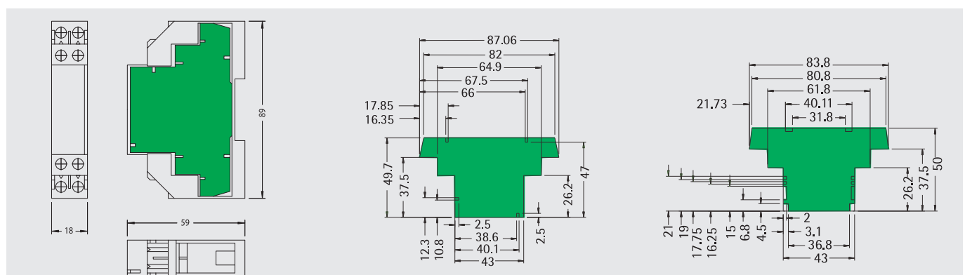
Abmessungen Grundgehäuse
